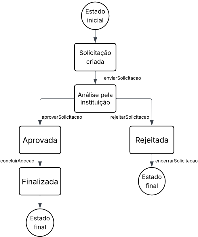
Diagrama de Estados (Solicitação de Adoção) - IPA-WZ
